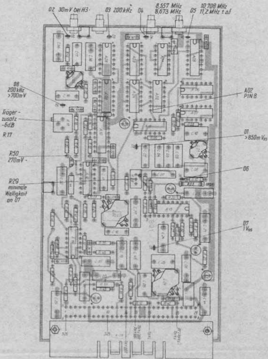
Leiterbild Bestockungsseite
