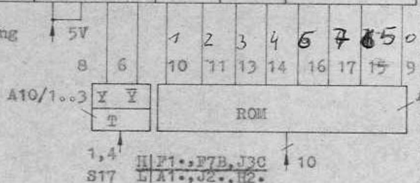
Bild 3 Programmierung und Beschaltung der Teiler-Kaskade A14, 15
