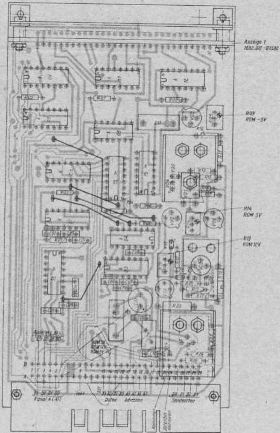
Leiterbild Bestückungsliste
