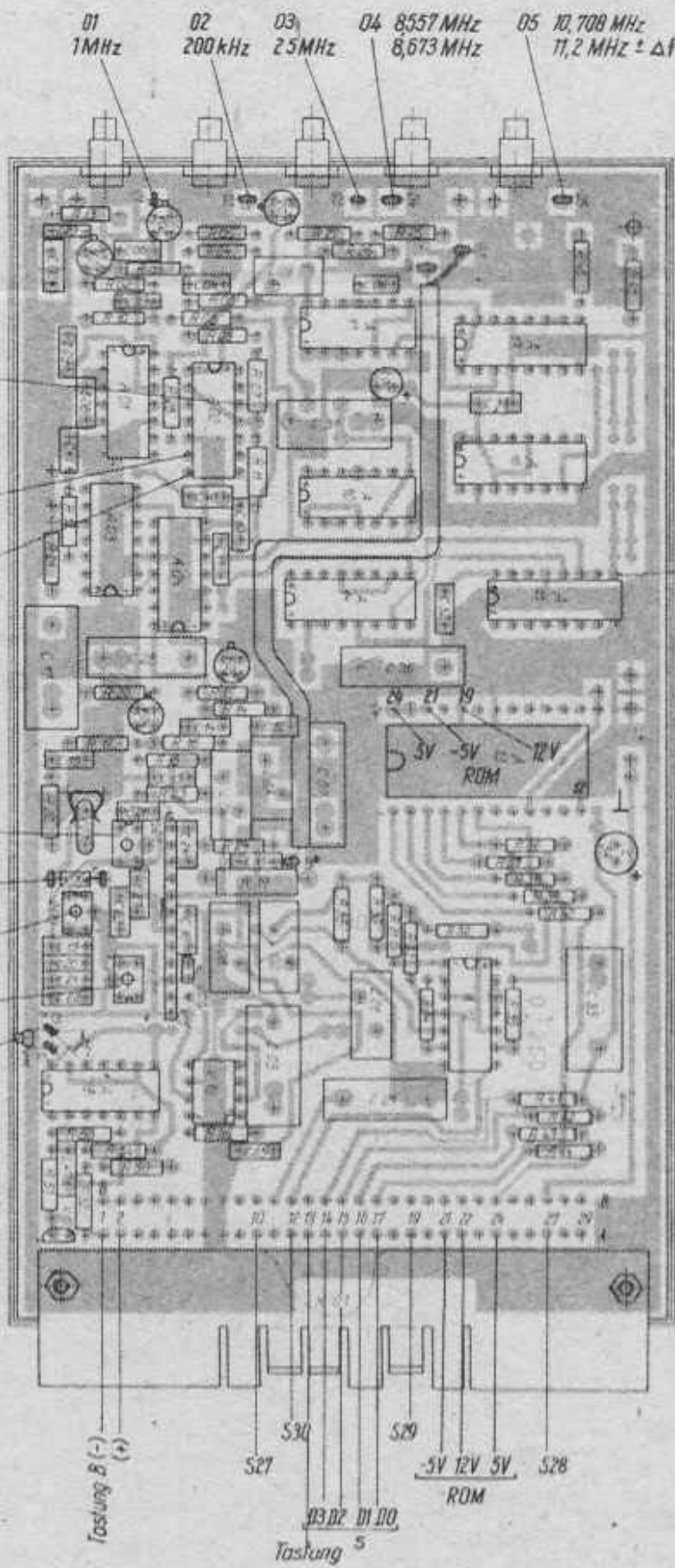
Leiterbild Bestückungsseite
