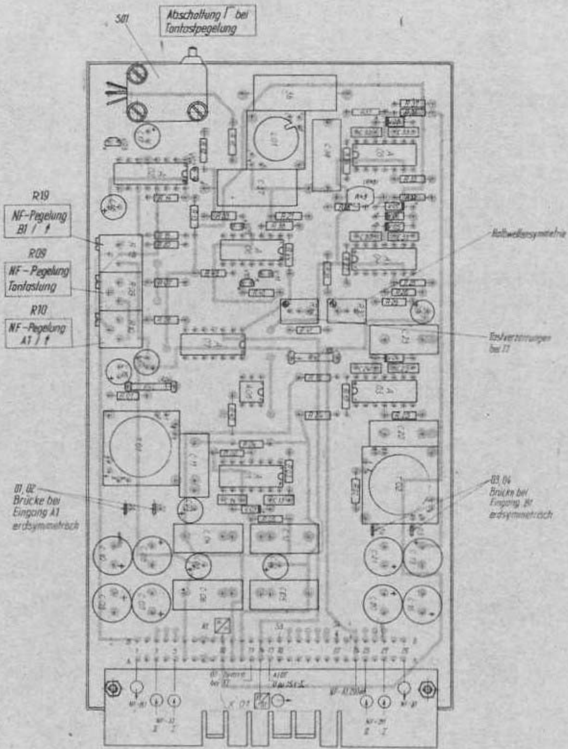
Leiterboard Bestückungsplan
