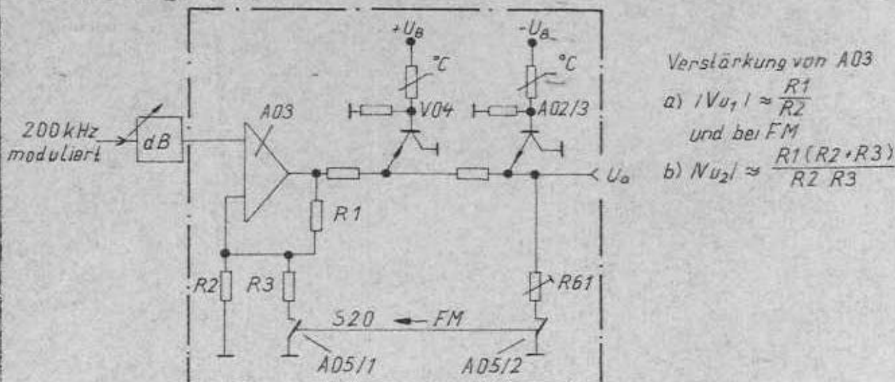
Bild 1 Begrenzeranordnung mit umschaltbarem Begrenzer-Einsatzpunkt
