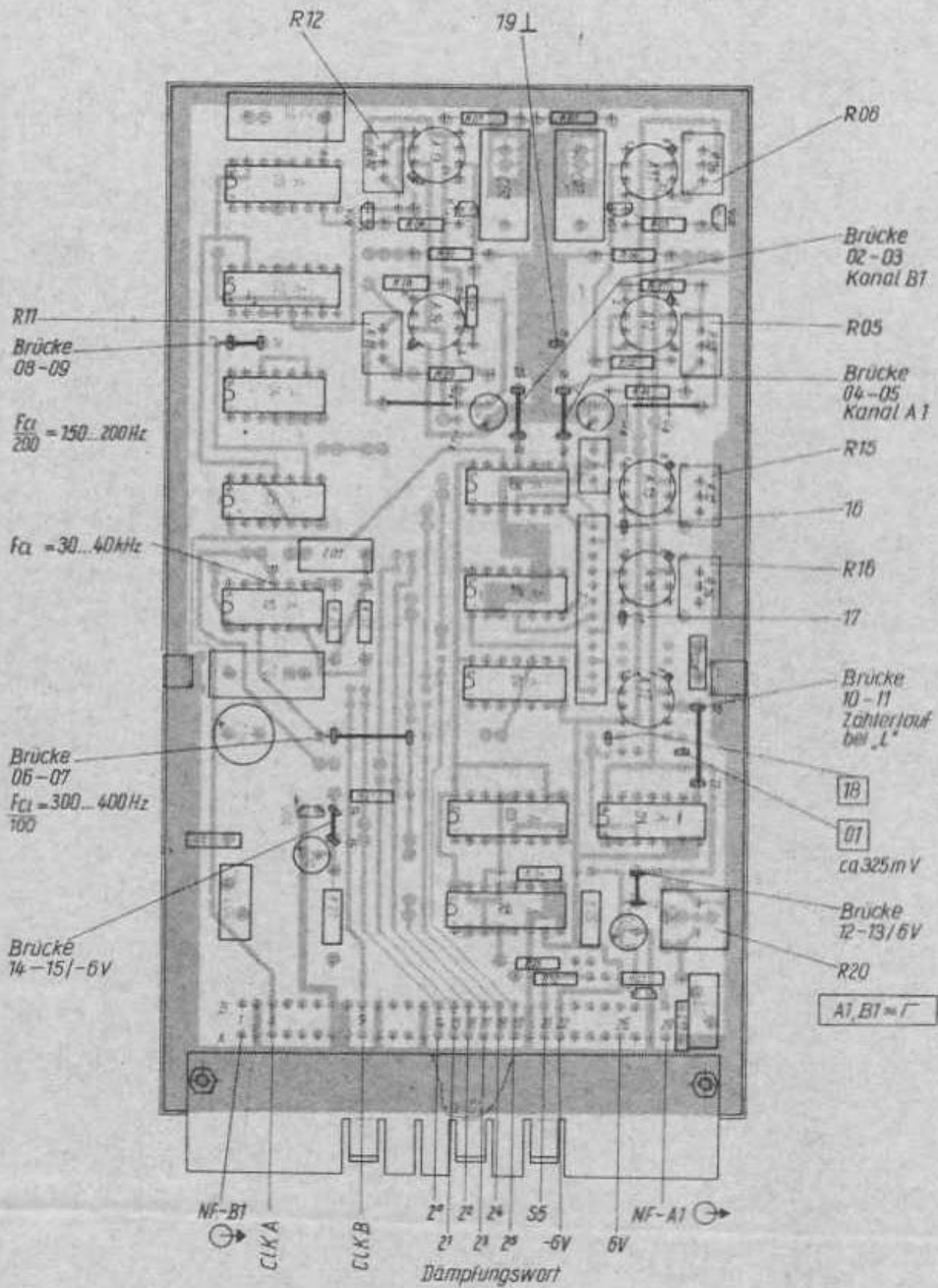
Leiterbild Bestückungsseite
